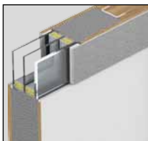
двукамерен стъклопакет, клас на противовзломност P4, рамкиран с неръждаема стомана.
