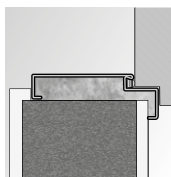
АГАТ Монтаж без анкерирани елементи
