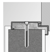
ОПАЛ Монтаж с дюбели
