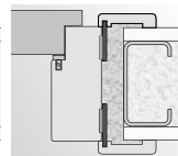
монтаж с пена в тухлена стена
