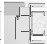
монтаж с болтове в стена от гипс-картон
