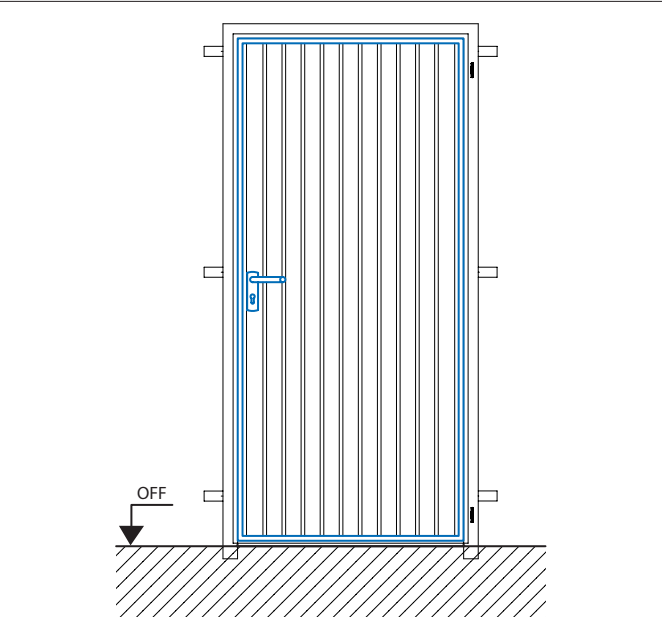
Einbau bei Außenanschlag
