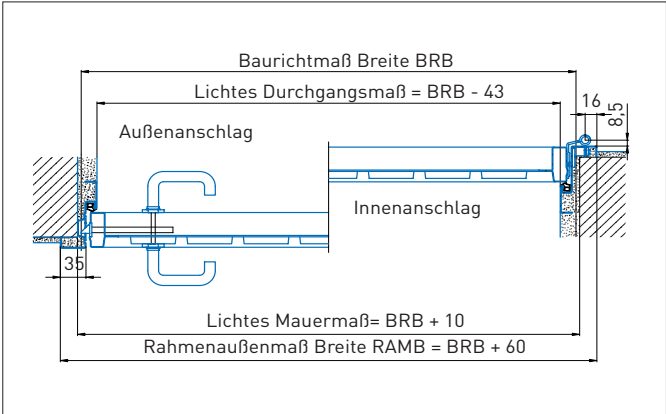
Einbau bei Innenanschlag
